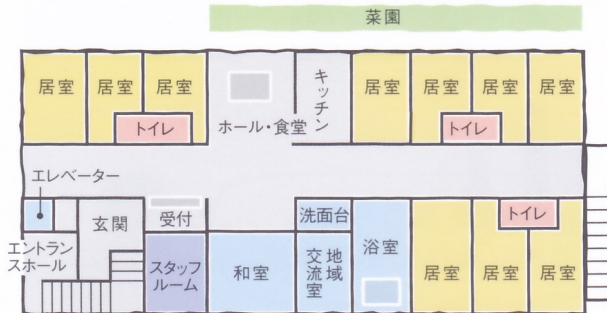
1階の平面図
